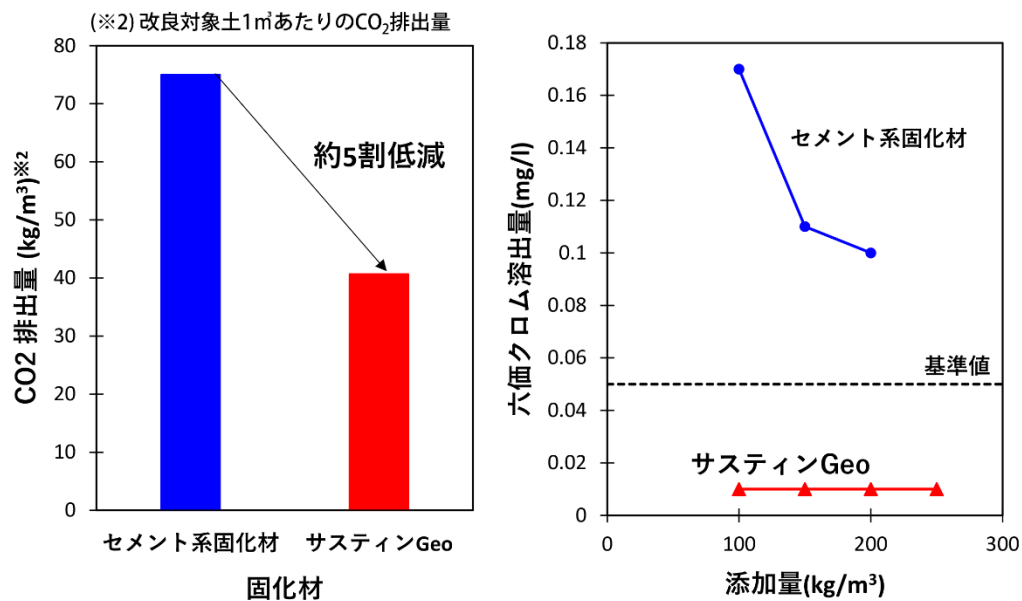
【CO 2 排出量と六価クロム溶出量の従来材料との比較】
