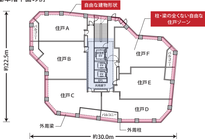
平面バリエーションの例
