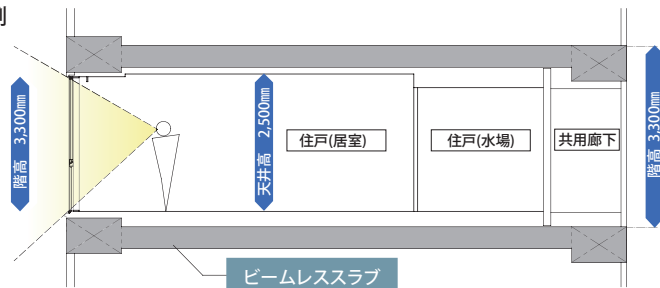
■住戸基準階平面の例
