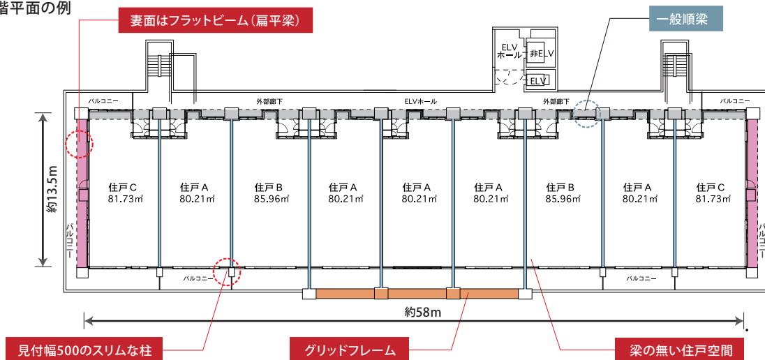
■基準階平面の例
