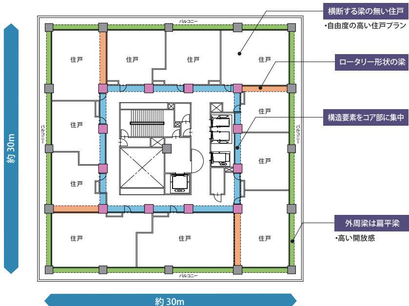
■住戸上層階平面の例
