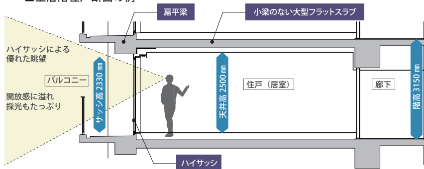
■上層階住戸断面の例
