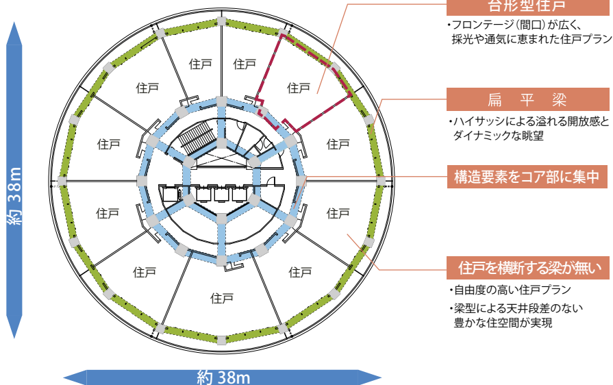
■住戸基準階平面の例
