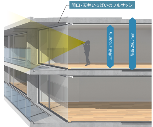
■バルコニー断面イメージ
