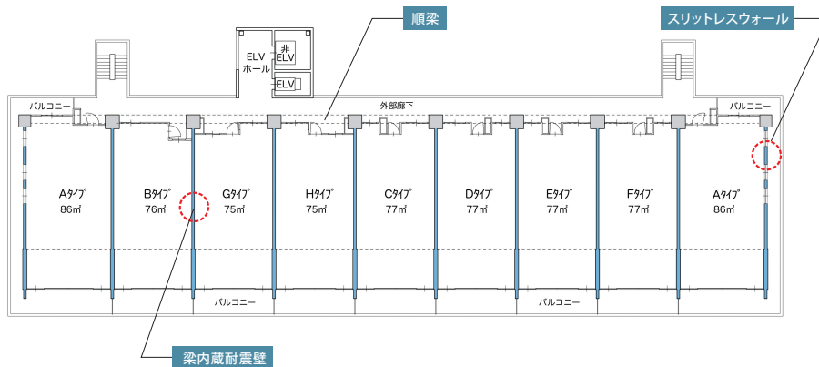
■基準階平面の例
