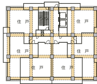
■従来の構造フレーム例
