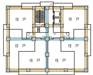
■Sulatto Compact Towerの 構造フレーム例
