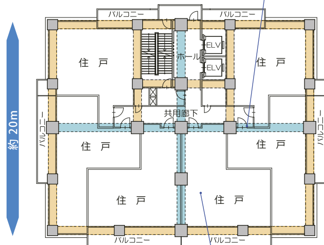
横断する梁を最少化した住戸
