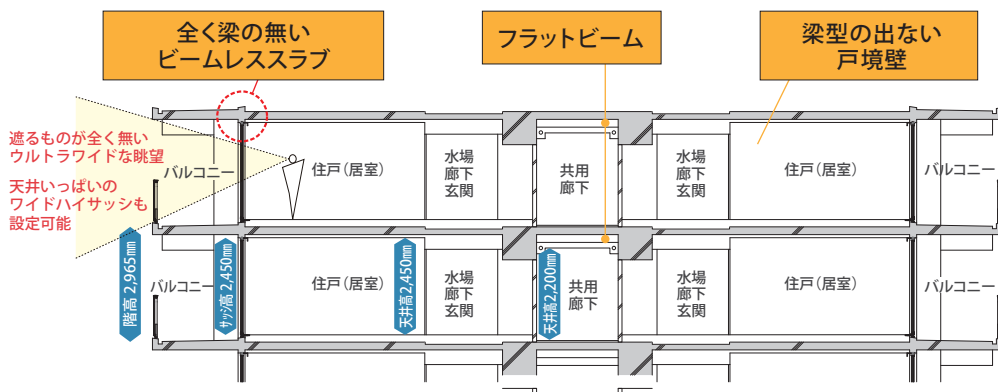
■住戸断面の例
