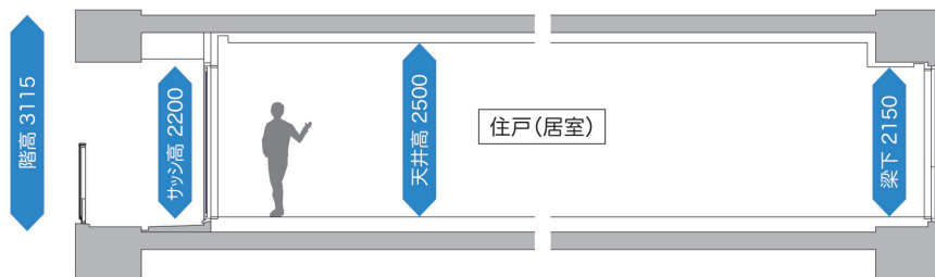
■住戸断面の例
